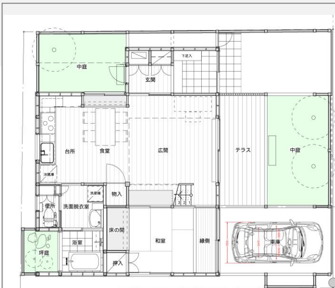
1階平面図
