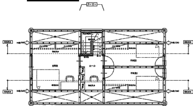
2階平面図
