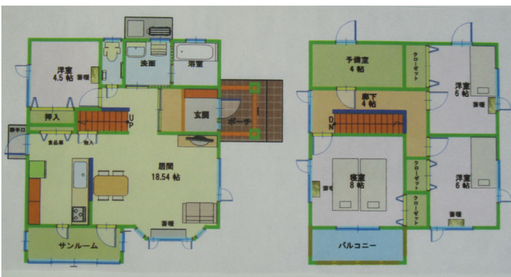
1階平面図
